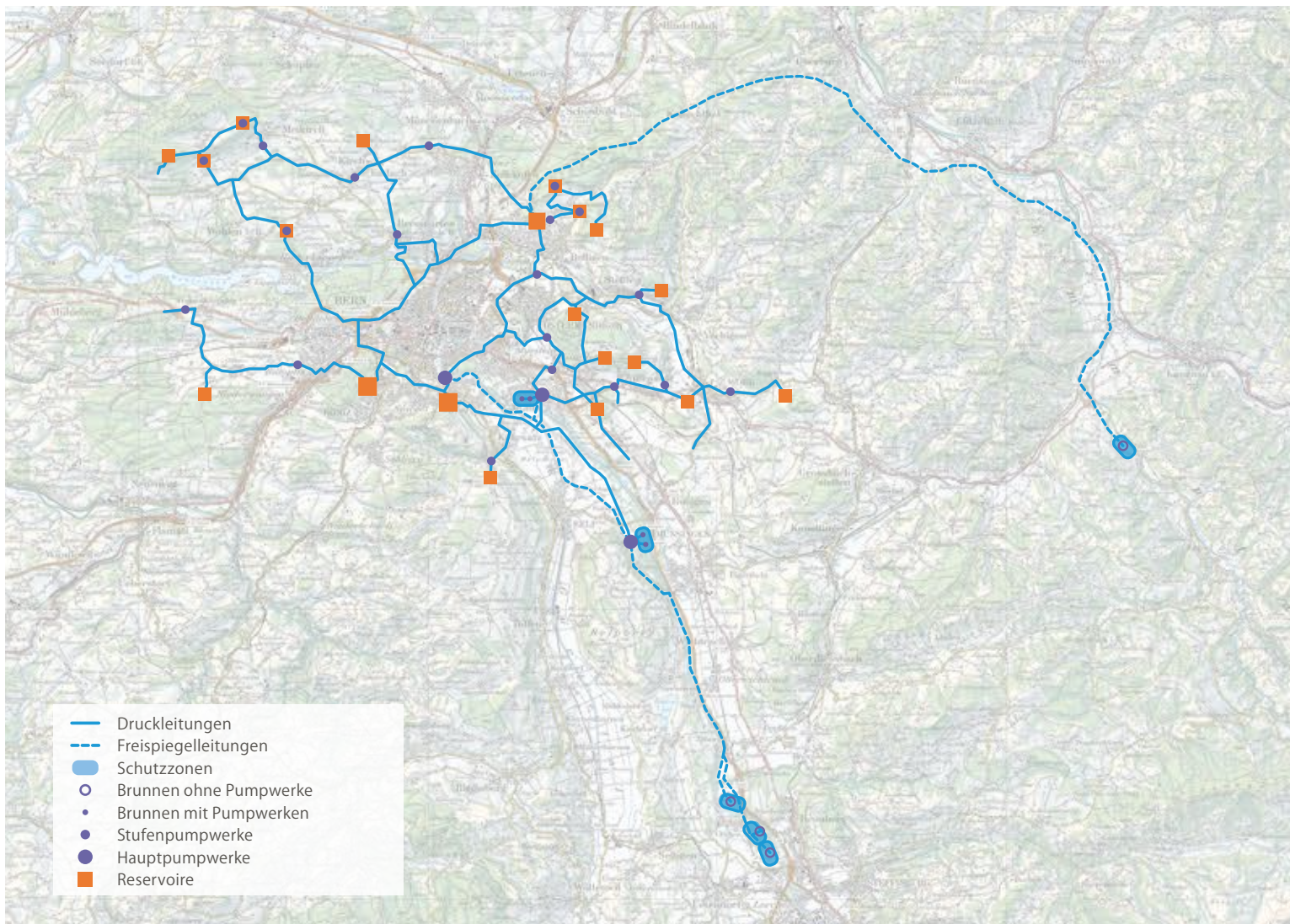
18 – Geografische Darstellung des Primärsystems der WVRB AG.
