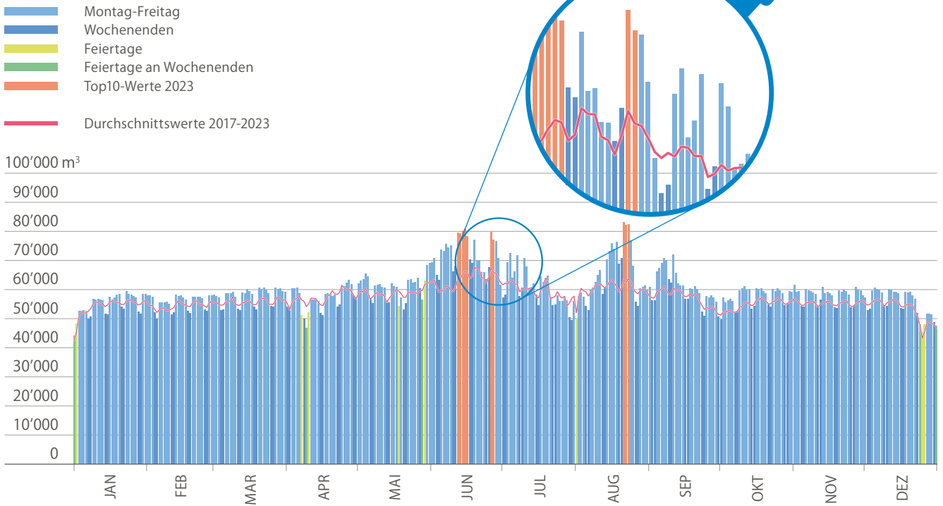
33 – Die tägliche Wasserabgabe 2023 und rot eingezeichnet das Mittel über 7 Jahre im Verbund.
