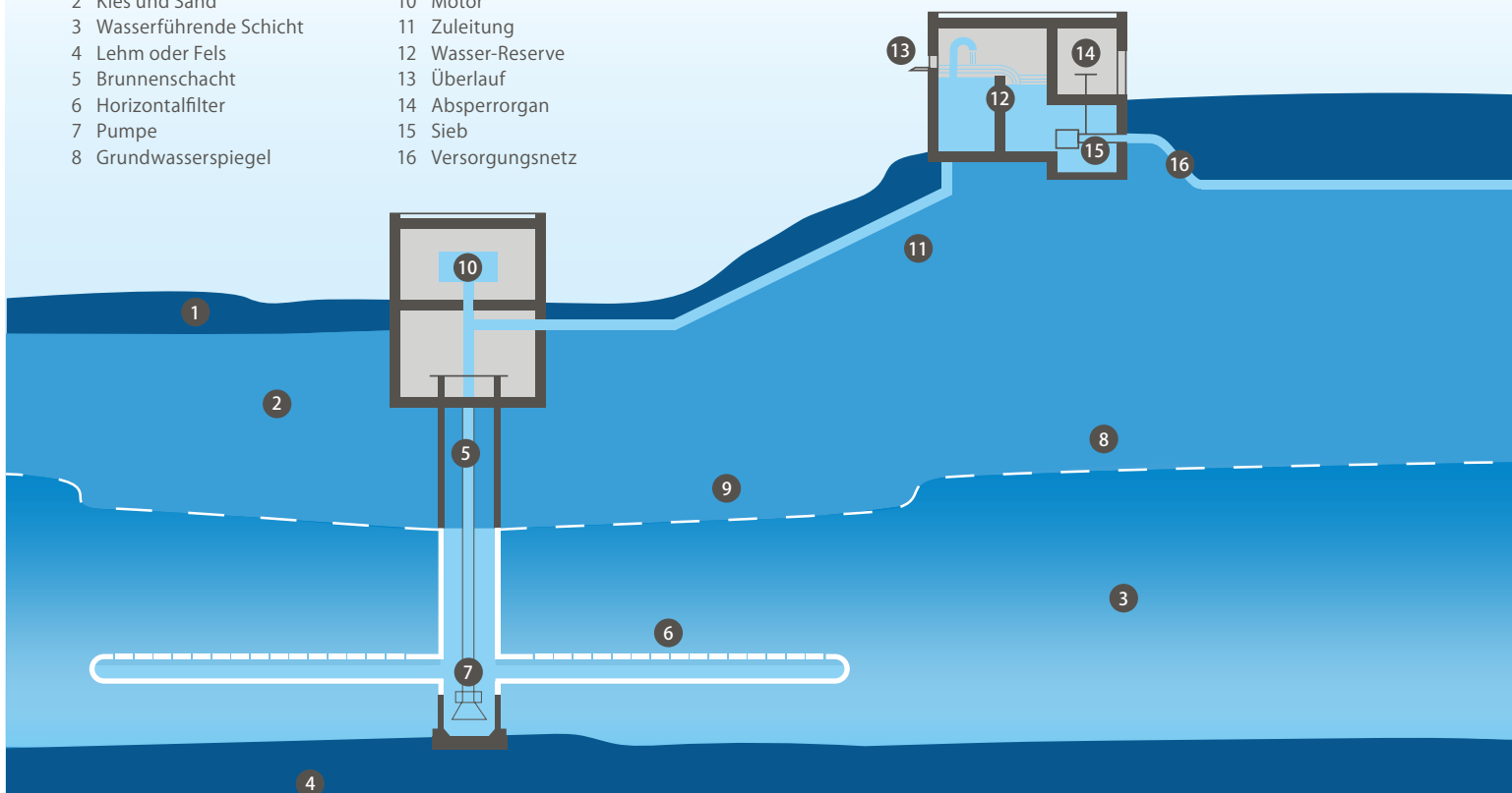
42 – Schematische Darstellung einer Grundwasserfassung inklusive Reservoir.
