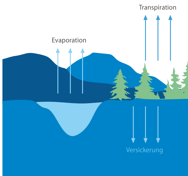
36 – Evapotranspiration ist die Summe aus der Transpiration und der Evaporation. Im Sommer gelangen nur wenige Niederschläge ins Grundwasser. Die wesentlichen Grundwasseranreicherungen finden meistens im Frühling statt.
