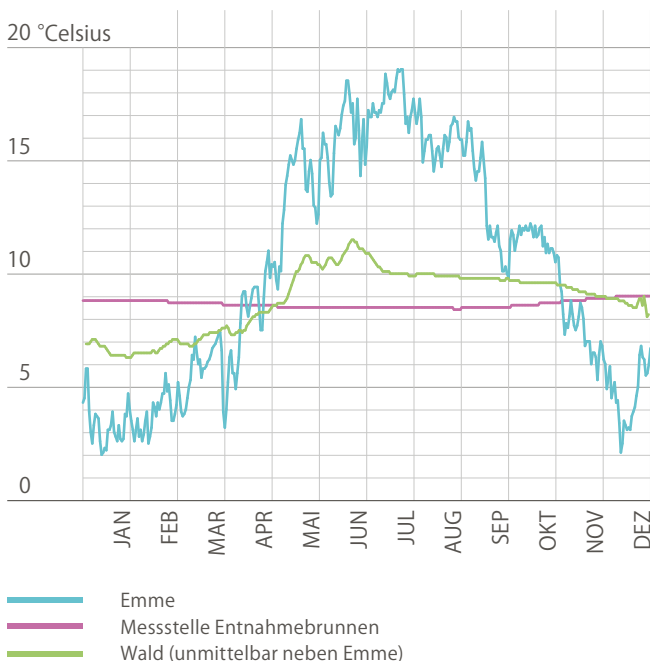
43 – Temperaturkurve der Wassertemperaturen in der Aeschau. Die Messwerte sind Tagesmittelwerte in der Emme, unmittelbar neben der Emme im Grundwasser und beim Entnahmebrunnen.
