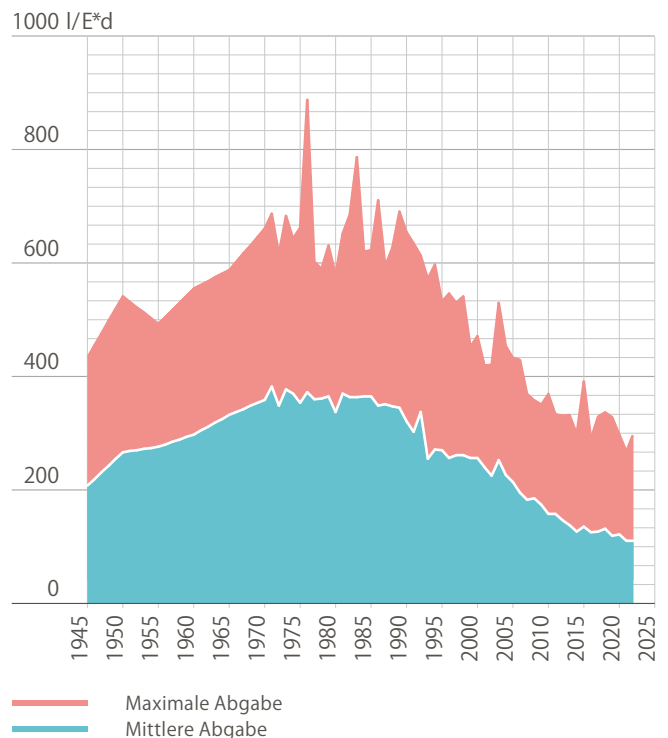
29 – Entwicklung des täglichen Trinkwasserverbrauchs pro Person und Tag in der Schweiz seit 1945. Entscheidend für die Dimensionierung der Wasserversorgung ist der Spitzenverbrauch.
