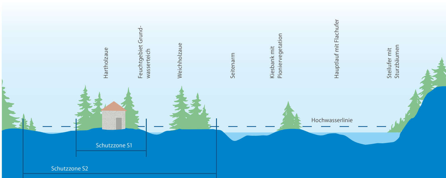
59 – Schematische Darstellung der Gefährdung des Trinkwassers durch Gewässer im Bereich der Schutz-zonen.
